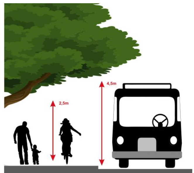
Lichtraumprofil (Quelle: BUND)
