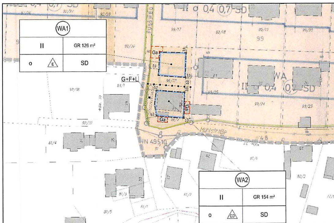
Abb. 6: Synopsenplan Bebauungsplan Nr. 3 „Hoffeld“ mit Einarbeitung der 3. Änderung
